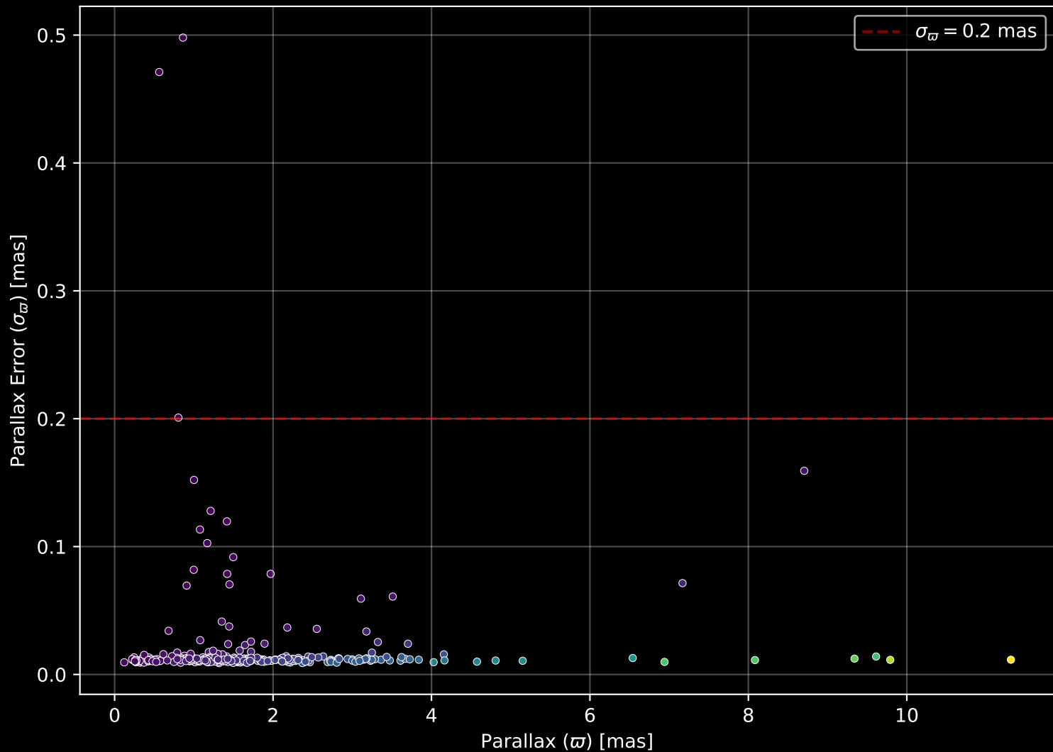
GALAH DR4 Field: [453] Parallax Quality (n= 299)
