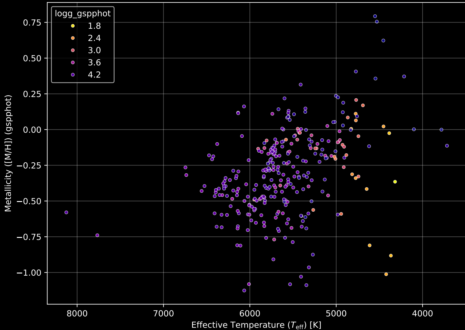
GALAH DR4 Field: [453] Stellar Population Parameters (n= 299)
